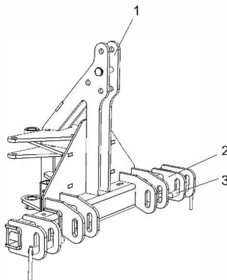
Illustration 6 Trepunktsbuk
