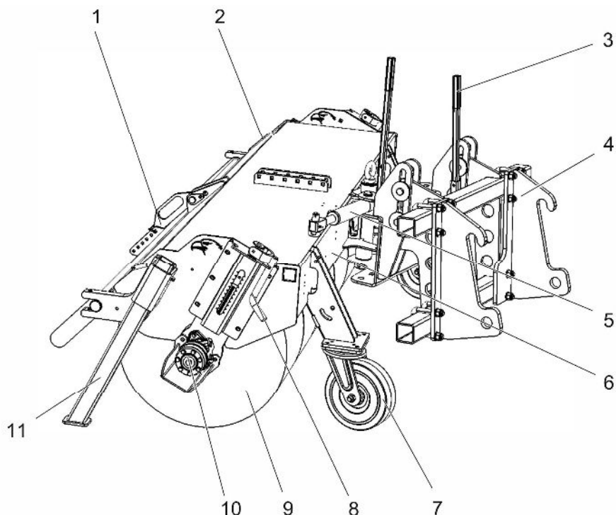
Illustration 2 Fejemaskine K 600
