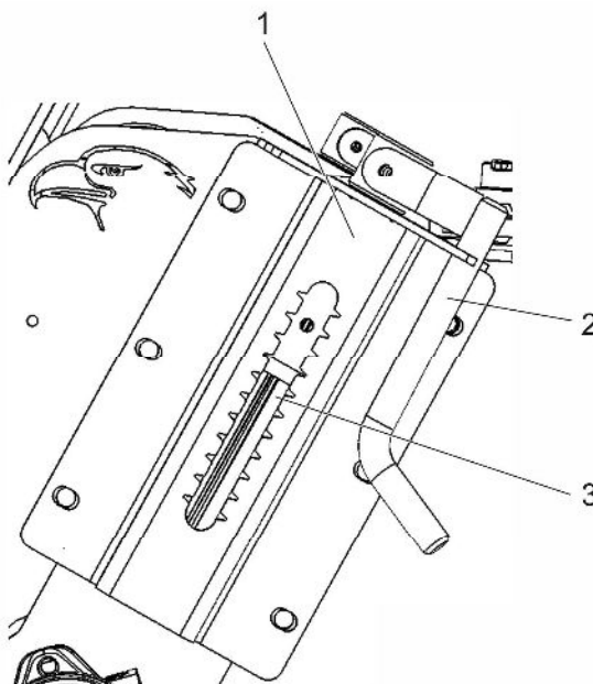
Illustration 15 Højdeindstilling fejervalse
